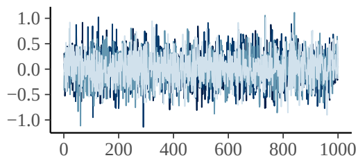
b_B_AUC.bl
