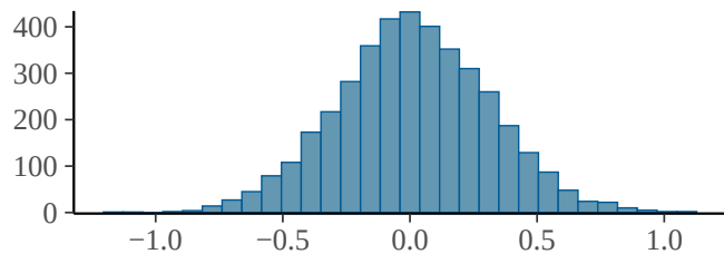
b_B_AUC.bl
